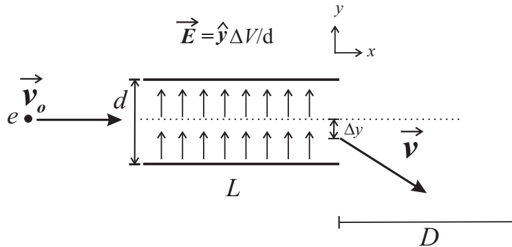
Figure 3: Déviation d'un électron par un champ électrostatique
