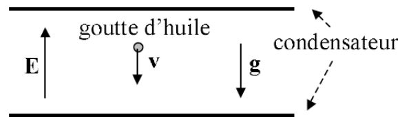
Figure 6: Expérience de Millikan
