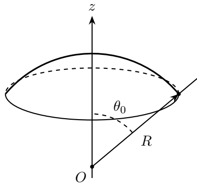
Figure 7: Calotte sphérique de centre O , de rayon R et d'angle \theta_0
