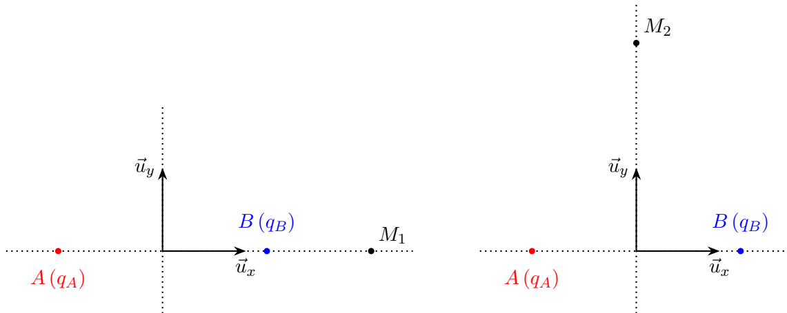
Figure 4: Dipôle électrique et points d'observation M_1 et M_2
