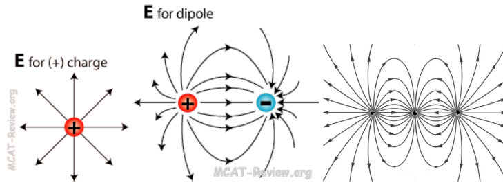
Figure 5: Champ et équipotentiels d'une charge, d'un dipôle et d'un quadrupôle électrique.
