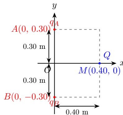
Figure 1: Deux charges sur l'axe Oy et une charge sur l'axe Ox
