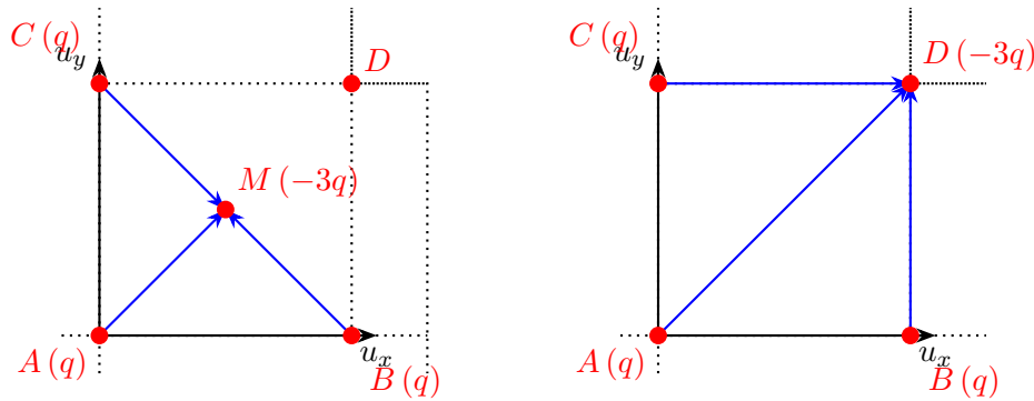
Figure 2: Position des charges dans le carré
