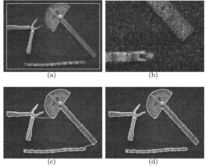
FIGURE 1 – Image réelle (386×533 pixels). (a) Initialisation. (b) Zoom sur un coin d'image. (c) Première étape de convergence. (d) Modification de la topologie.
