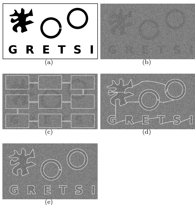
FIGURE 2 – Image synthétique (350×600 pixels). (a) Vérité terrain. (b) Image bruitée. (c) Initialisation. (d) Première étape de convergence. (e) Modification de la topologie.
